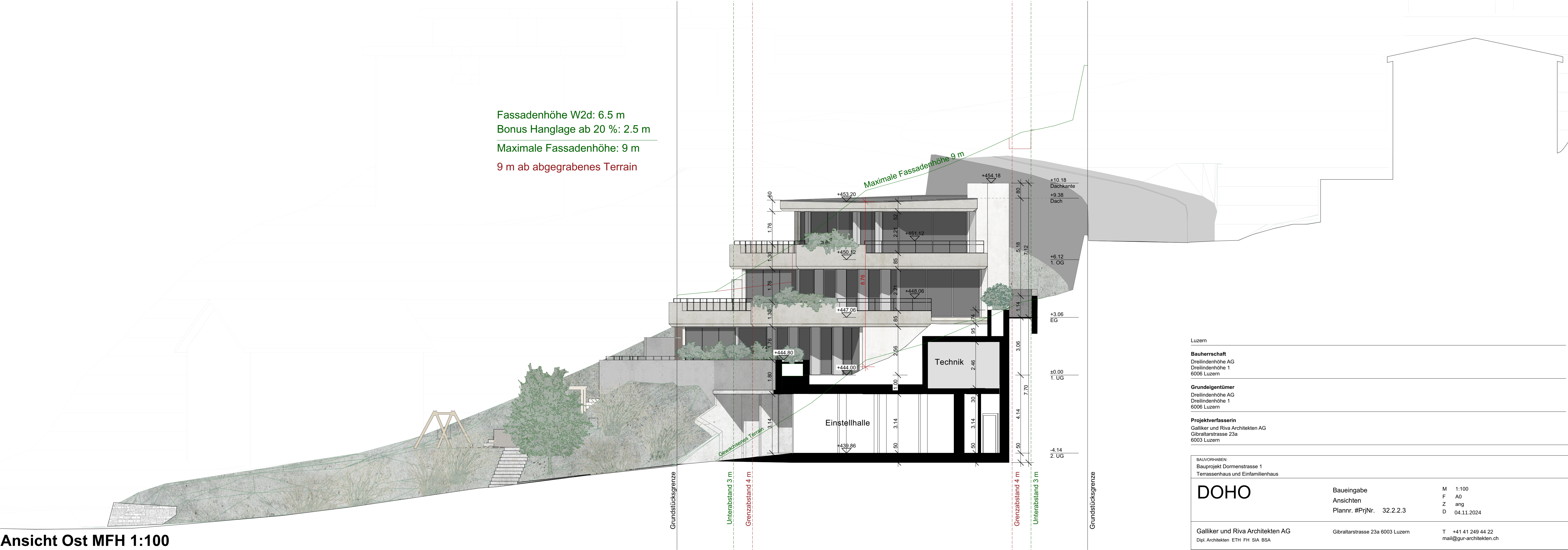
Ansicht Ost MFH 1:100
