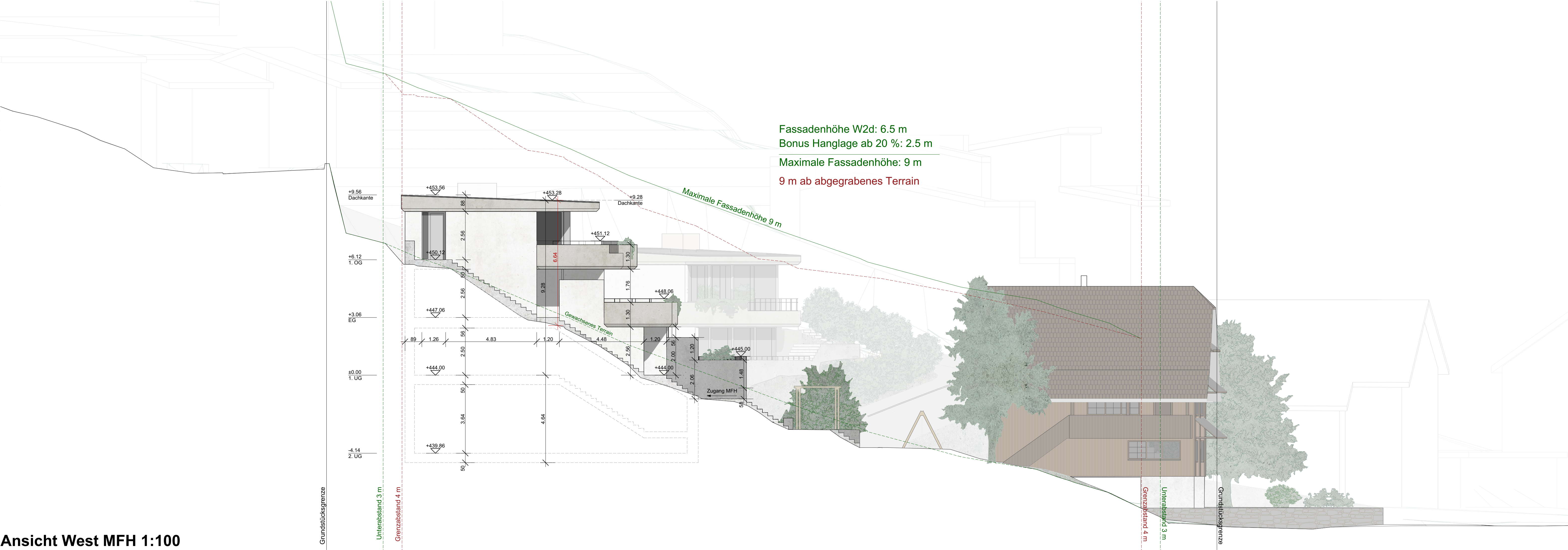
Ansicht West MFH 1:100
