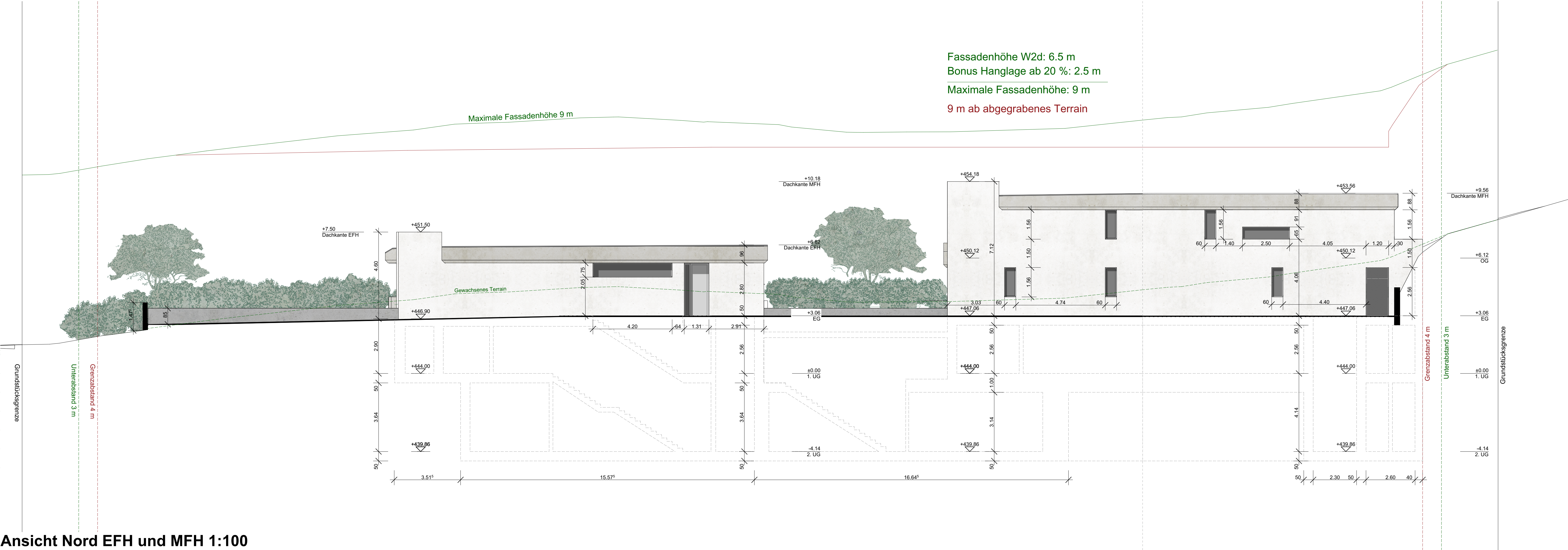
Ansicht Nord EFH und MFH 1:100
